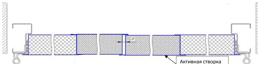
Горизонтальный разрез ворот (схема)
